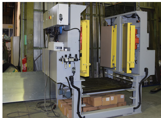
Système de placage octabin, conçu et réalisé par Meca ei pour optimiser le conditionnement de polystyrène
